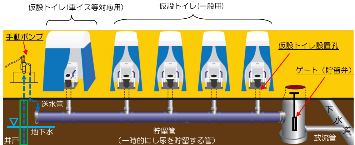
災害用トイレシステム概要図
